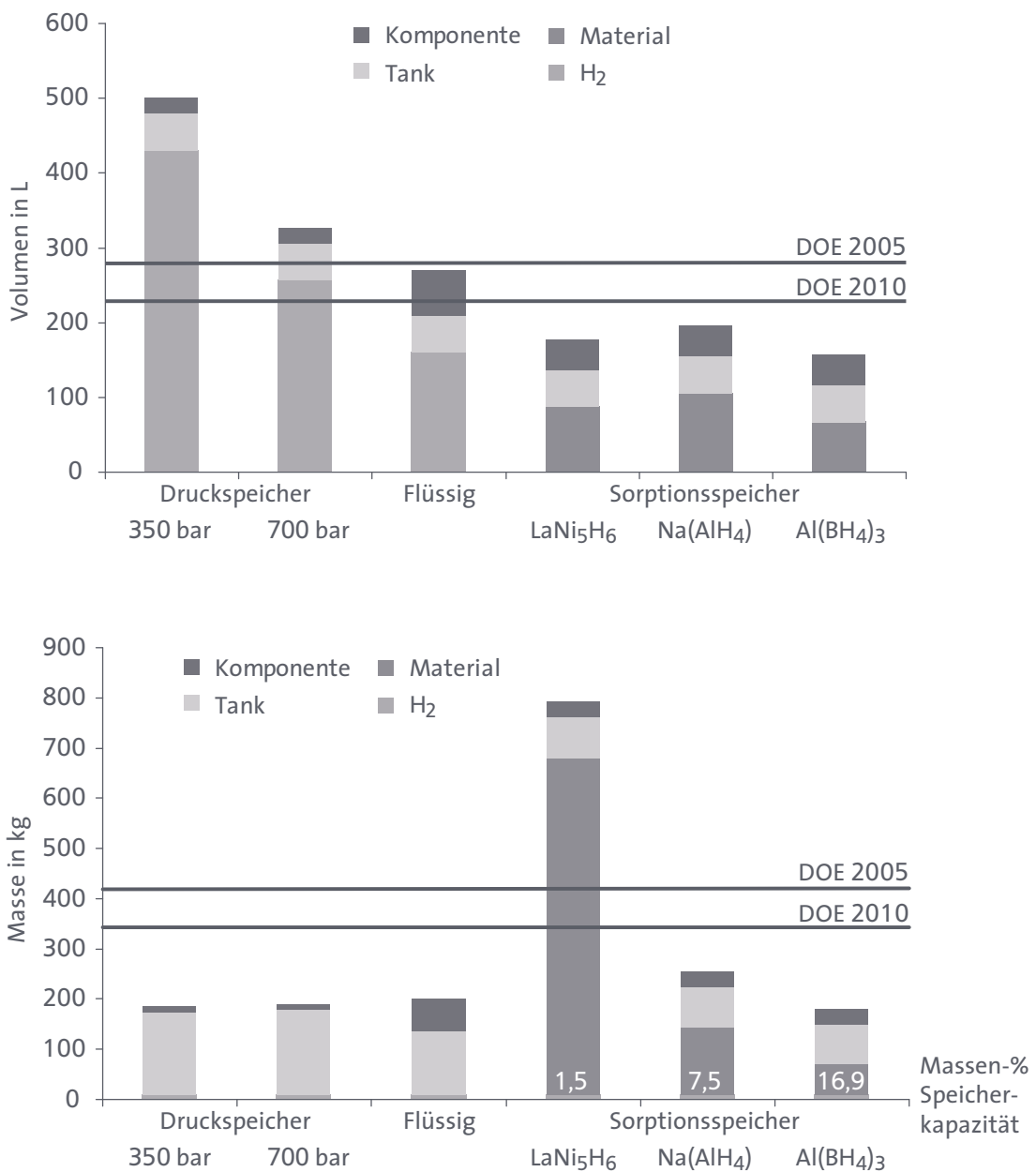
ABB. 7 VERGLEICH VON WASSERSTOFFSPEICHERTECHNOLOGIEN NACH VOLUMEN (OBEN) UND NACH MASSE (UNTEN) DES SPEICHERTANKS (10 KG H 2 FÜR 700 KM REICHWEITE)
