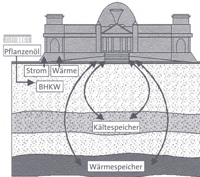
ABB. 2 ENERGIEKONZEPT* DES REICHSTAGSGEBÄUDES (SCHEMATISCH)
