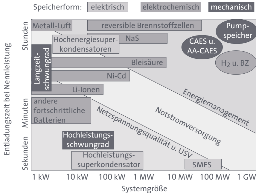
ENERGIESPEICHERSYSTEME FÜR STATIONÄRE EINSATZGEBIETE
