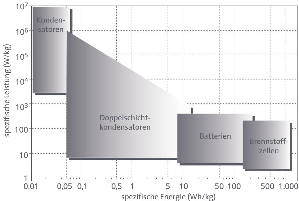
ABB. 9 RELATION ZWISCHEN SPEZIFISCHER LEISTUNG UND SPEZIFISCHER ENERGIE VERSCHIEDENER SPEICHERSYSTEME (RAGONE-PLOT)
