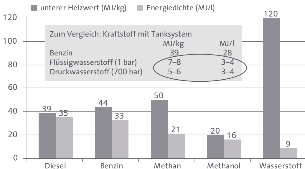
ABB. 5 BEWERTUNG DER SPEICHERDICHTEN VON KRAFTSTOFFEN OHNE TANKSYSTEM
