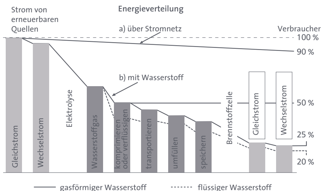
ABB. 11 ENERGIEVERLUSTE BEI DER NUTZUNG VON WASSERSTOFF ALS ZWISCHENSPEICHER FÜR ELEKTRISCHEN STROM
