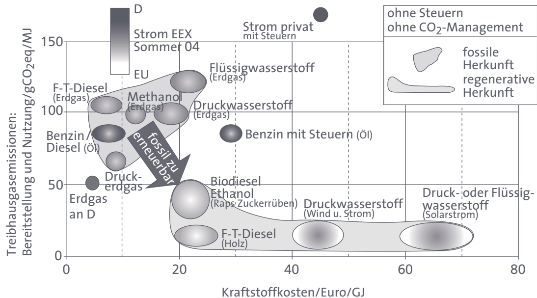
ABB. 6 GEGENÜBERSTELLUNG VON BEREITSTELLUNGSKOSTEN UND KLIMAGASEMISSIONEN VON KRAFTSTOFFEN (KLIMAGASEMISSIONEN INKLUSIVE DER VOLLSTÄNDIGEN VERBRENNUNG VON JEWEILS 1 MJ)
