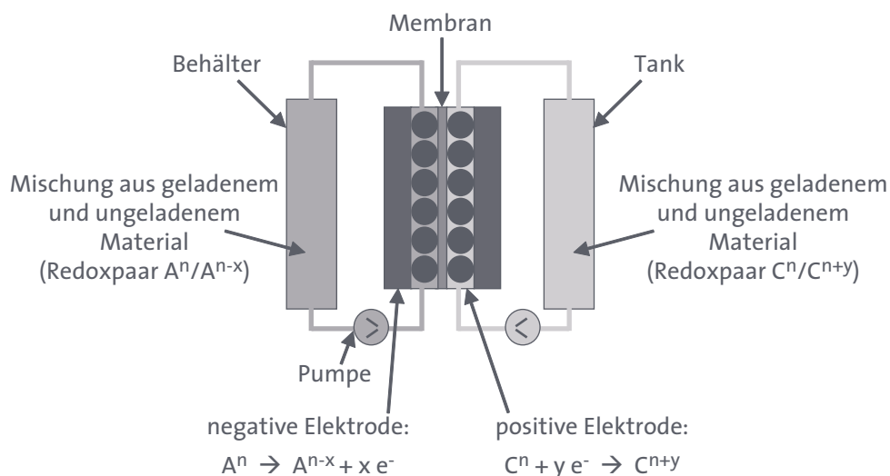
AUFBAU EINER REDOX-FLOW-BATTERIE
