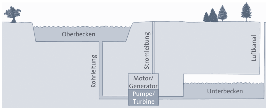
ABB. 1 FUNKTIONSPRINZIP EINES UNTERIRDISCHEN PUMPSPEICHERKRAFTWERKS
