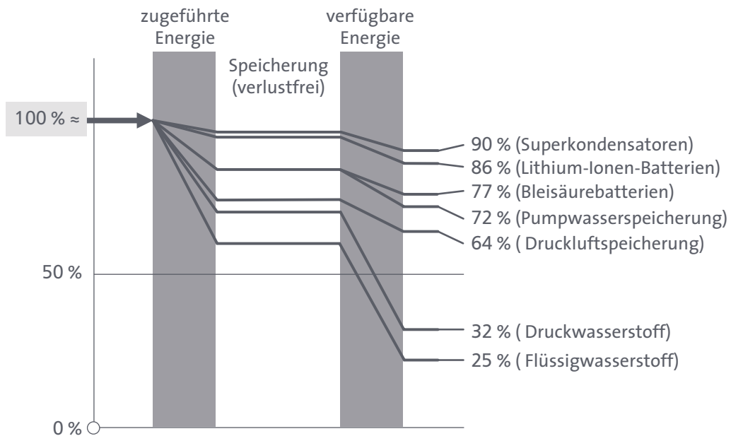
ABB. 12 UMWANDLUNGSVERLUSTE VERSCHIEDENER SPEICHERMÖGLICHKEITEN
