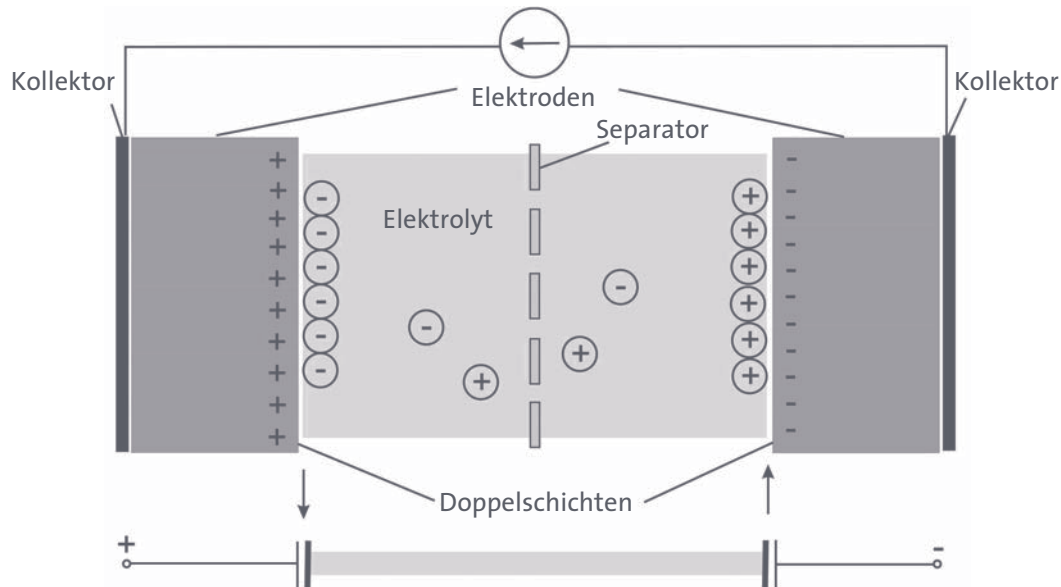
ABB. 8 PRINZIPSKIZZE EINES ELEKTROCHEMISCHEN KONDENSATORS
