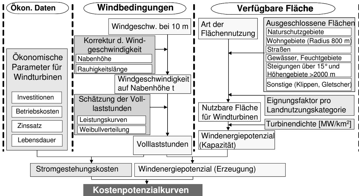
Abbildung 1: Schematische Darstellung der angewandten Methodik zur Bestimmung der Kostenpotenzialkurven für Windstrom (Onshore)
