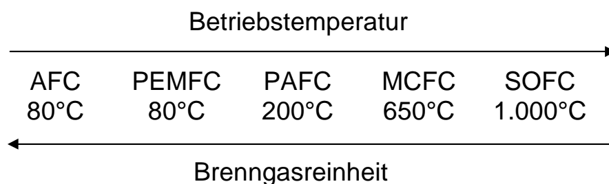
Abb. 7: Zusammenhang zwischen Betriebstemperatur der Brennstoffzelle und geforderter Brennstoffreinheit
