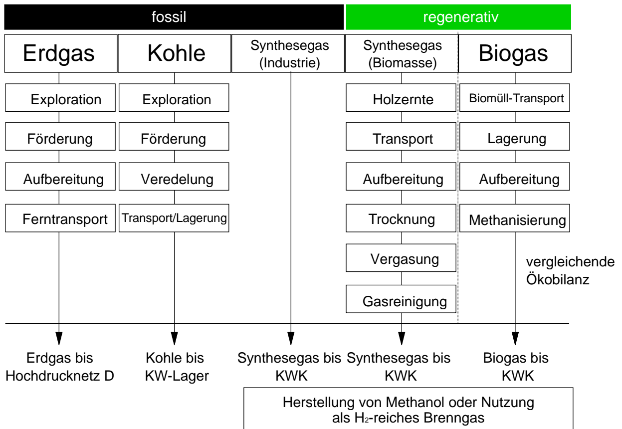
Abb. 42: Analysierte Energieketten für industrielle und öffentliche Stromversorgung bis zur "Schnittstelle Nutzer"
