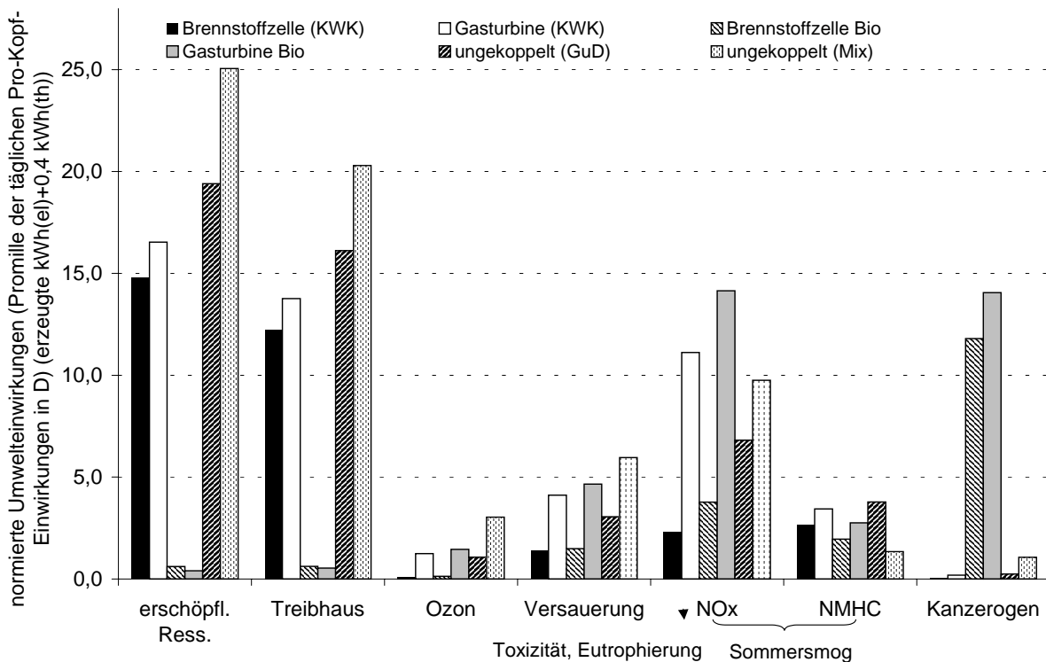
Abb. 48: Umwelteinwirkungen der industriellen Kraft-Wärme-Kopplung im Vergleich zur ungekoppelten Stromerzeugung bezogen auf die jährlichen Pro-Kopf-Einwirkungen in Deutschland für das Jahr 2010
