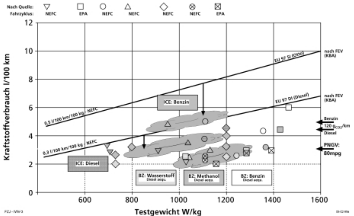
Abb. 10: Kraftstoffverbrauch ( I_{\text{Benzin}}/100 \text{ km} beziehungsweise I_{\text{Diesel}}/100 \text{ km} ) für Verbrennungsmotoren (ICE) und für Brennstoffzelle ( \text{H}_2 , Methanol, Benzin) als Funktion des Testgewichts (Pkw)
