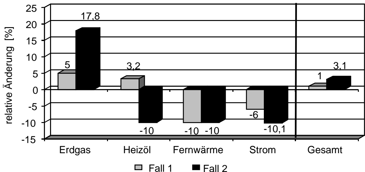
Abb. 37: Relative Änderung der Energieträgerstruktur des Sektors Haushalte bei 10%iger Implementierung von Brennstoffzellen-BHKW in Bezug auf die Trendskizze (Prognos/EWI 1998) (Deutschland, 2010)
