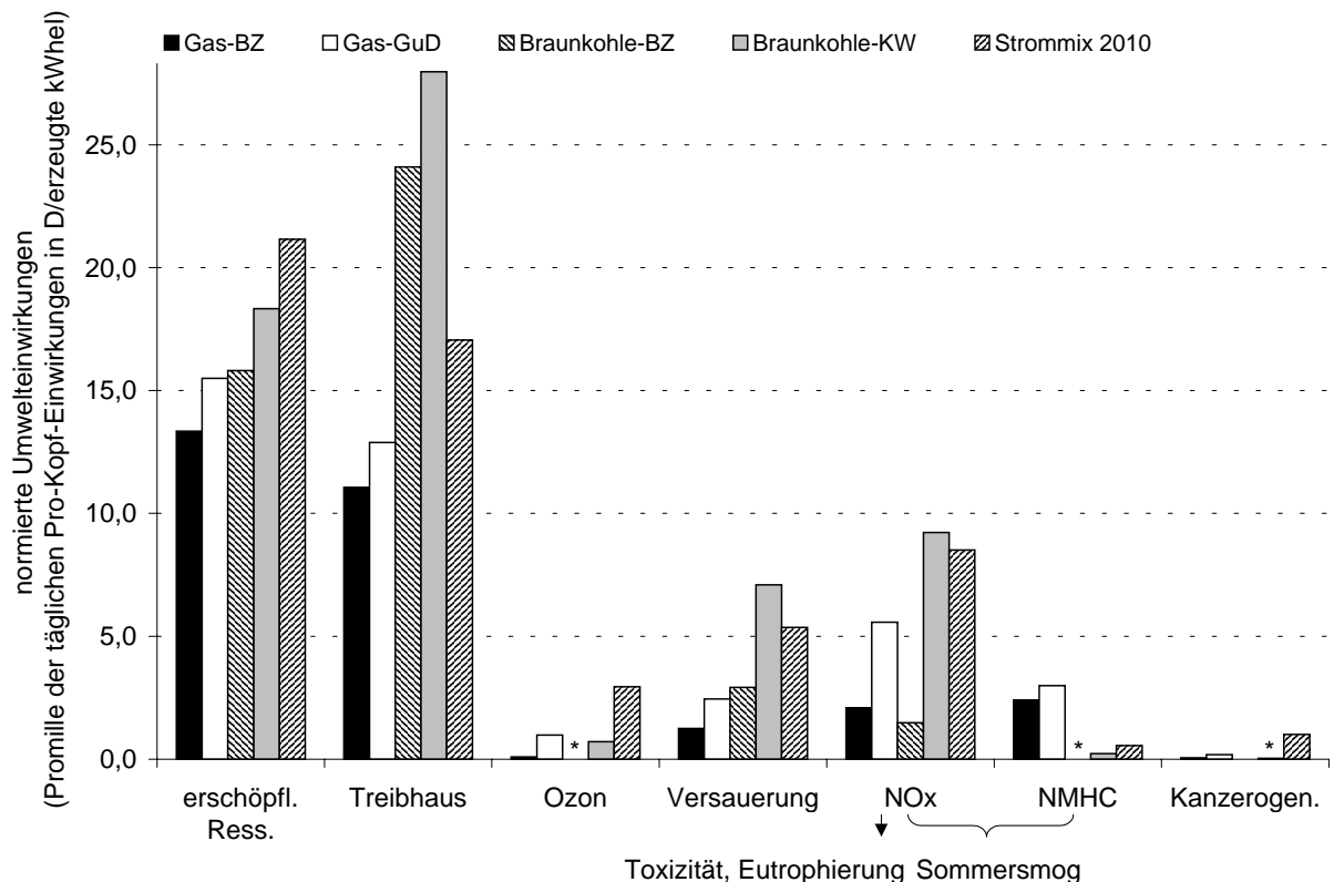
Abb. 50: Umwelteinwirkungen der ungekoppelten Stromerzeugung bezogen auf die jährlichen Pro-Kopf-Einwirkungen in Deutschland
