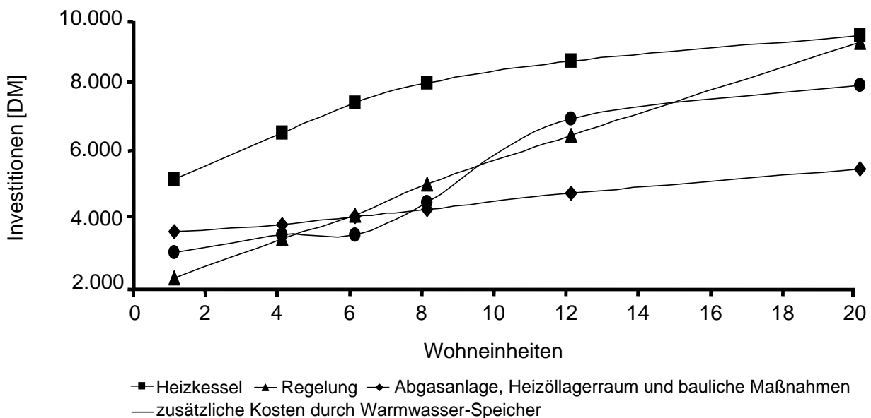
Abb. 29: Abhängigkeit der Investitionen für Erdgas-Brennwert-Heizungssysteme von der Gebäudegröße
