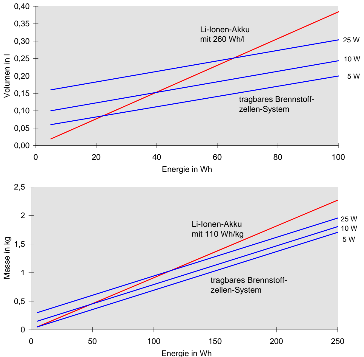
Abb. 56: Volumen und Gewicht eines tragbaren Brennstoffzellen-Systems in Abhängigkeit von der Kapazität
