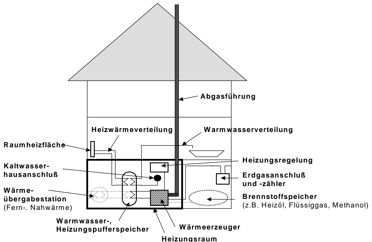
Abb. 23: Hauptkomponenten von Heizungssystemen (Erdgas, Heizöl, Fernwärme)
