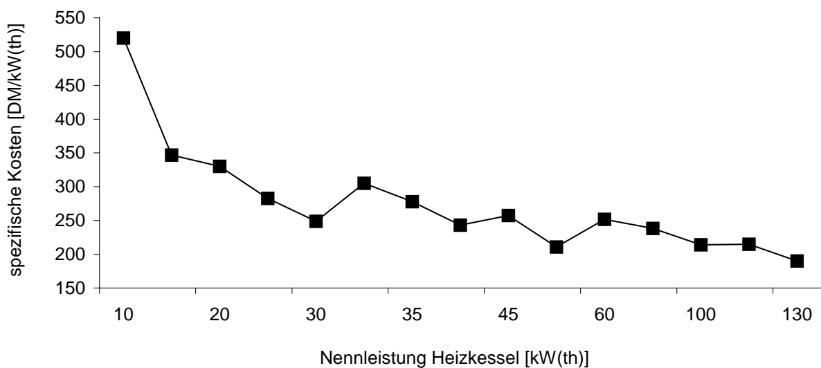
Abb. 31: Spezifische Kosten von Erdgas-Brennwertheizkesseln als Funktion der Nennleistung
