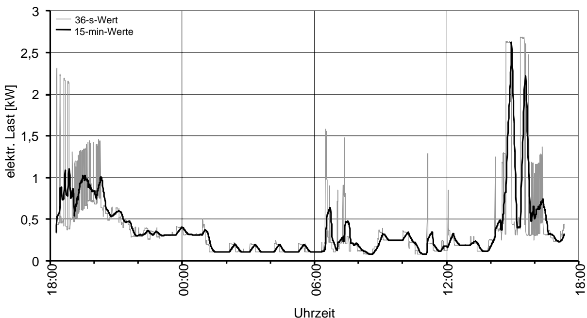
Abb. 26: Exemplarische Darstellung des Lastganges eines Einfamilienhauses (36-sec-Messwerte und 15-min-Mittelwerte)
