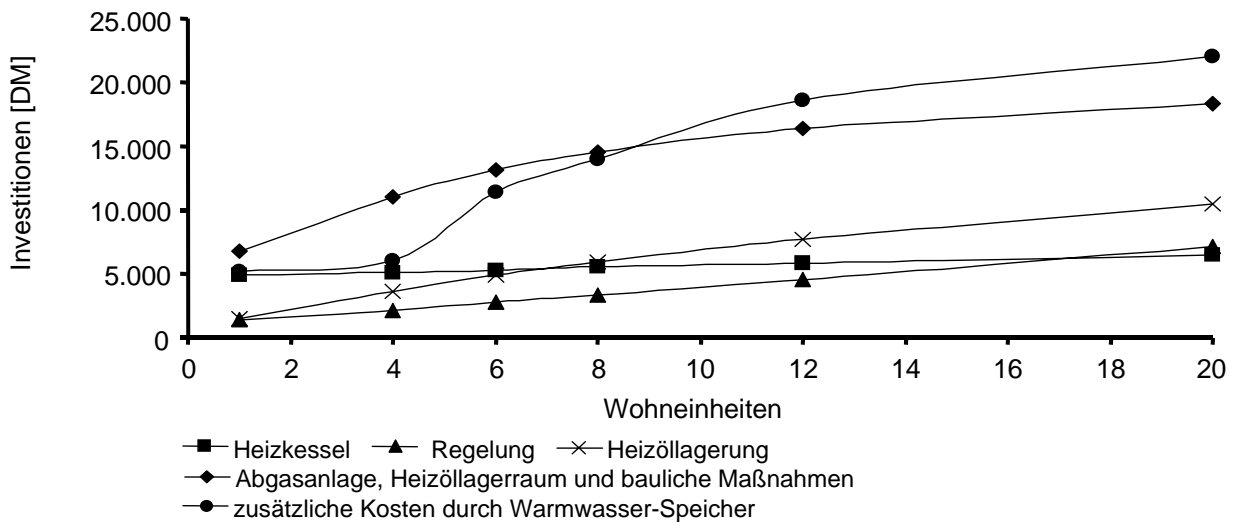
Abb. 30: Abhängigkeit der Investitionen für Heizöl-Niedertemperatur-Heizungssysteme von der Gebäudegröße
