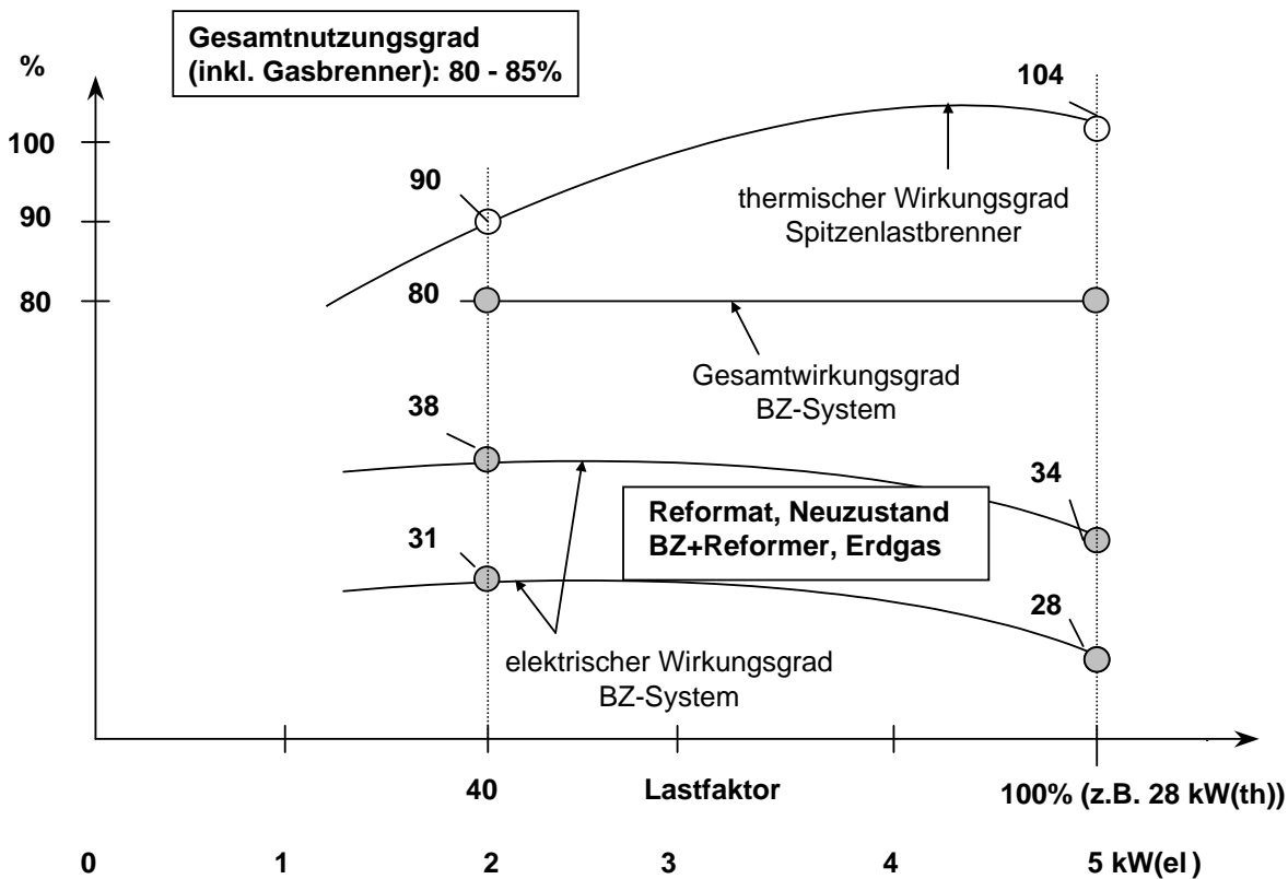
Abb. 28: Wirkungsgrade eines erdgasbetriebenen Brennstoffzellen-BHKW mit einem Erdgas-Brennwert-Heizkessel
