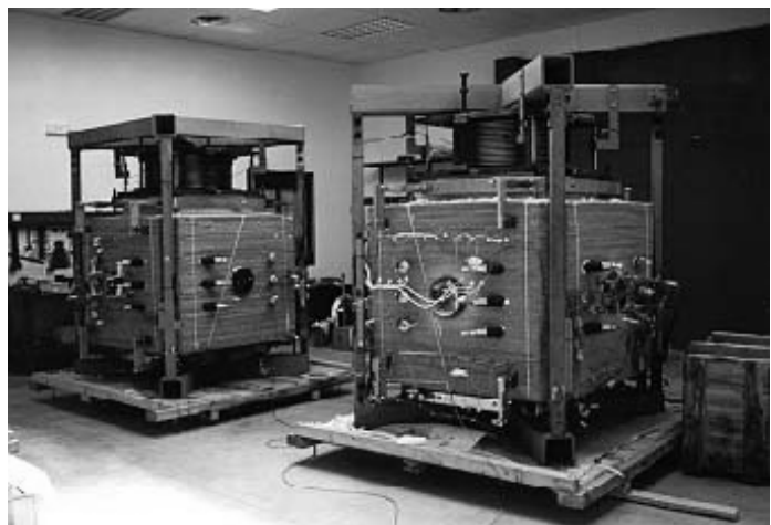
Abb. 5: Beispiele für technisch realisierte Brennstoffzellen-Stacks, hier von DeNora (links) und Ansaldo (rechts)
