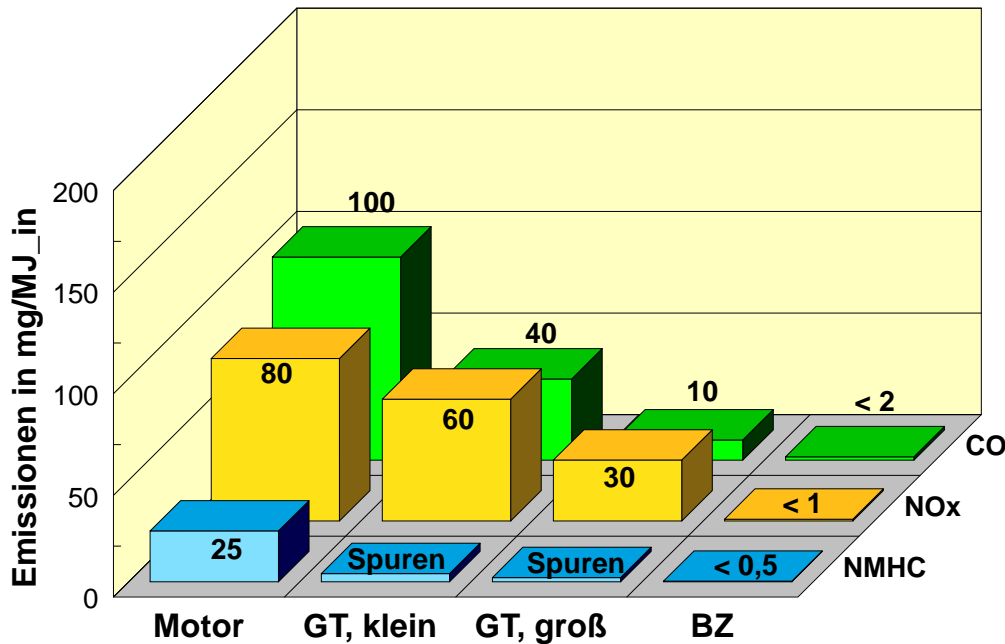
Abb. 45: Abschätzung von lokal freigesetzten Emissionen einzelner Anlagen für das Jahr 2010
