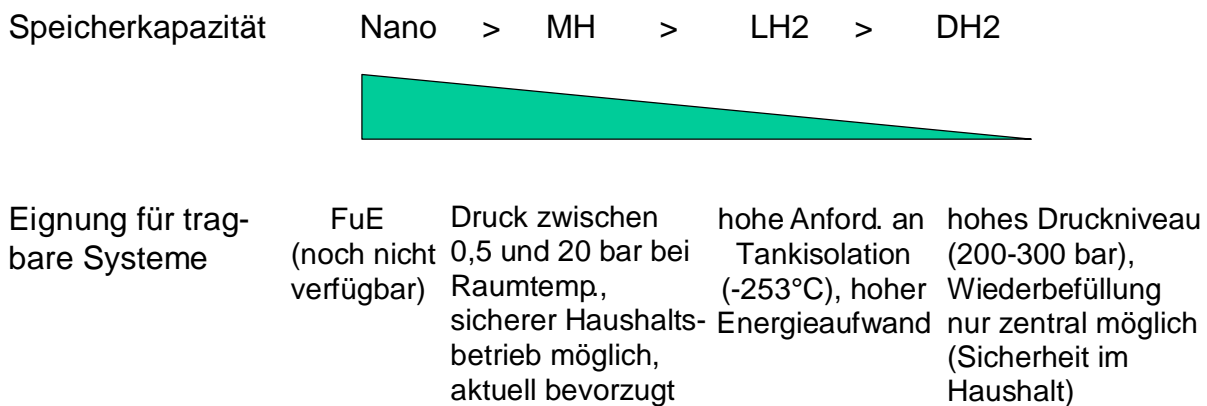
Abb. 54: Wasserstoff-Speicher für tragbare Brennstoffzellen-Systeme
