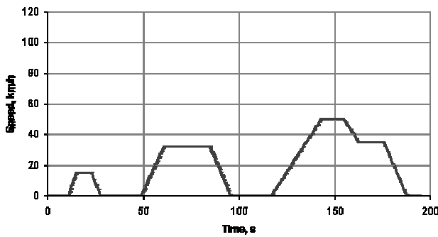
ECE-Zyklus
