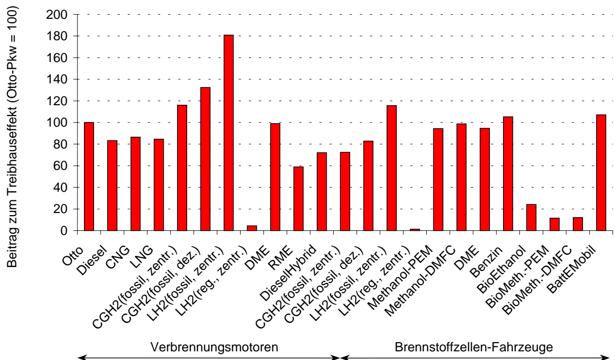
Abb. 11: Vergleich des Beitrages zum Treibhauseffekt*
