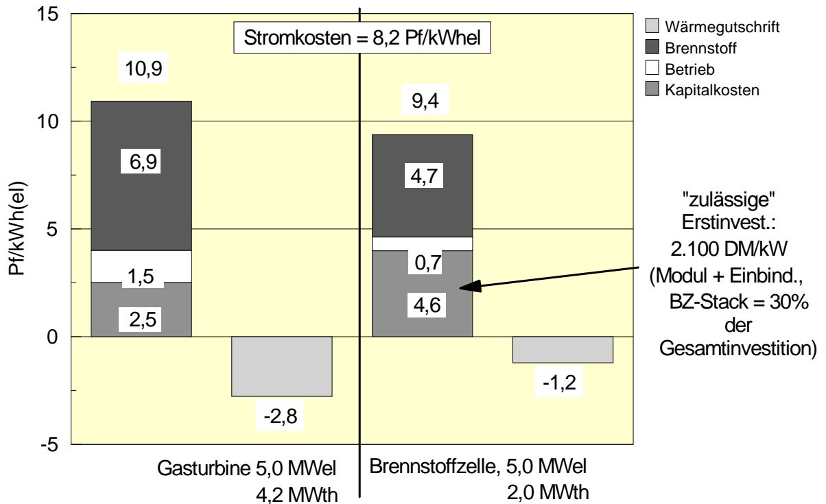
Abb. 44: Kostenstruktur (bezogen auf die Stromerzeugung) des Hybrid- und des Gasturbinen-Systems (5 MW (el)) bei gleichen Stromgestehungskosten
