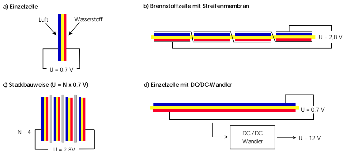
Abb. 53: Konzepte zur räumlichen Anordnung von Brennstoffzellen
