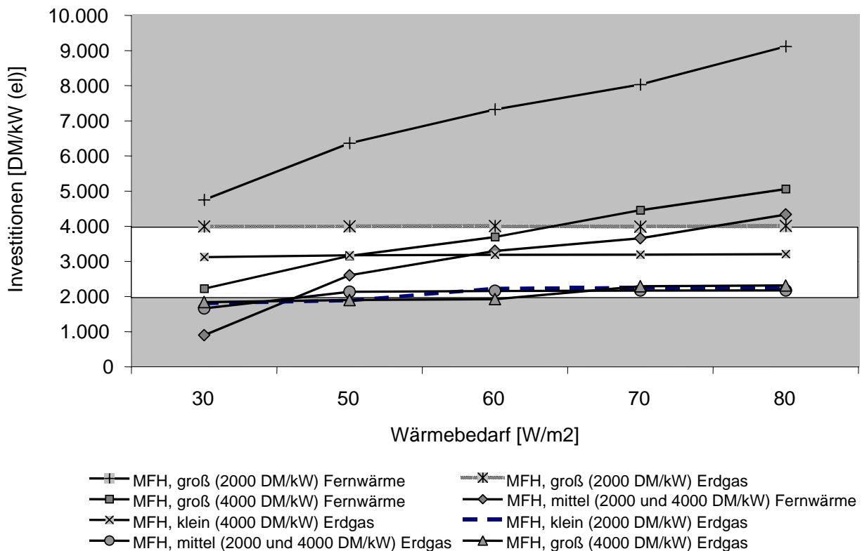
Abb. 36: Zulässige Investitionen (mit MWSt) der Brennstoffzellen-BHKW für die Varianten 1 und 4 (Darstellung praxisrelevanter Fälle)
