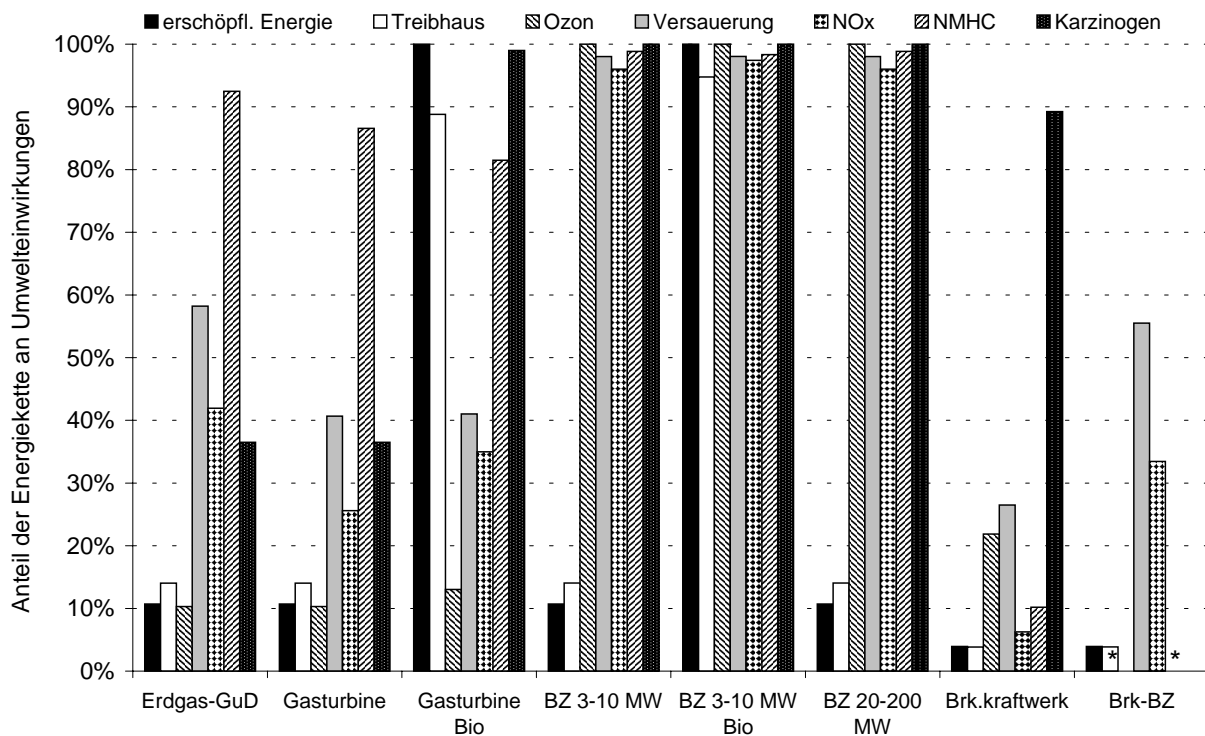
Abb. 52: Einfluss der vorgelagerten Brennstoff-Energieketten für die Umwelteinwirkungen bei einzelnen Technologien
