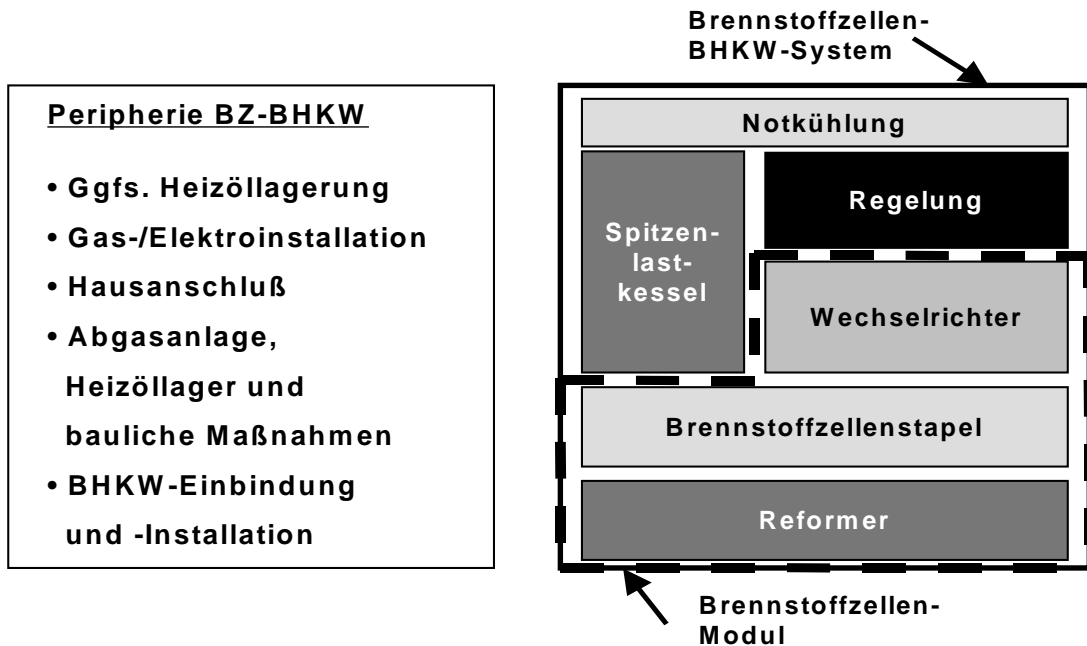
Abb. 32: Komponenten des Brennstoffzellen-Systems für die Kostenbetrachtung
