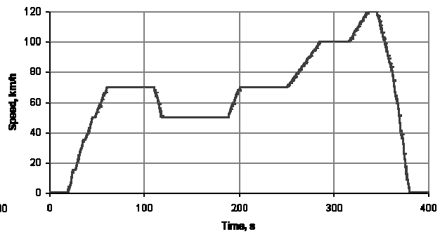
EUDC
