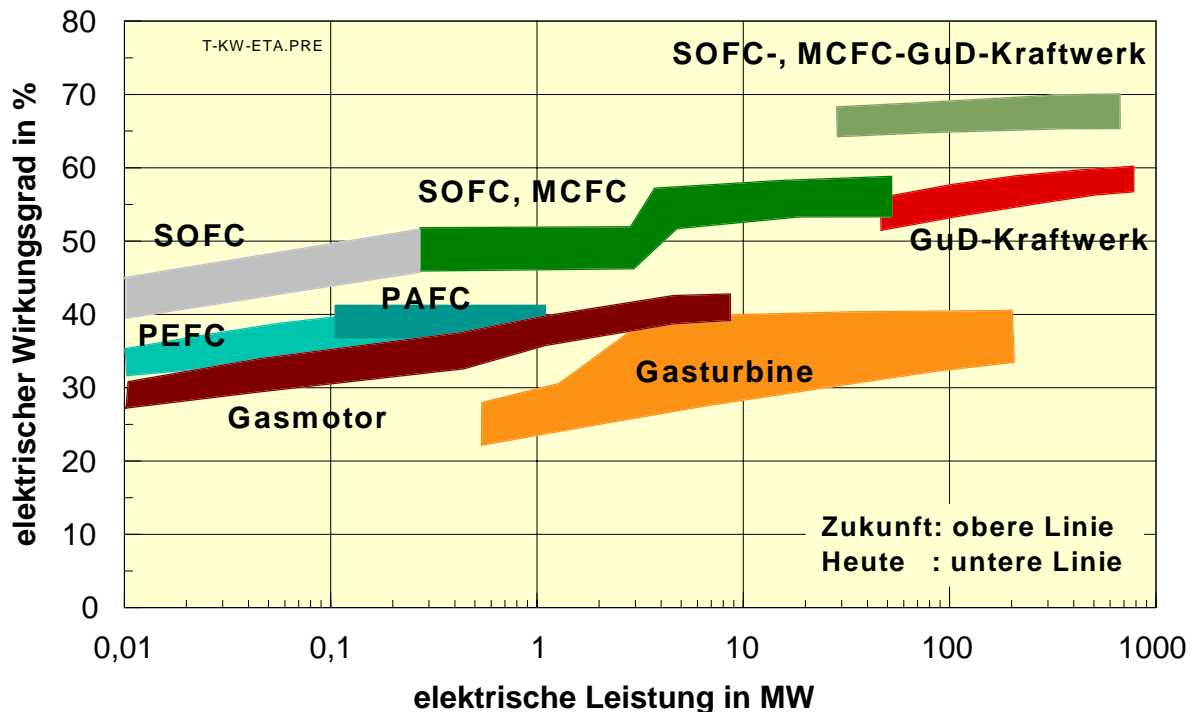
Abb. 43: Heutige und zukünftige elektrische Wirkungsgrade von Kraftwerken auf Erdgasbasis
