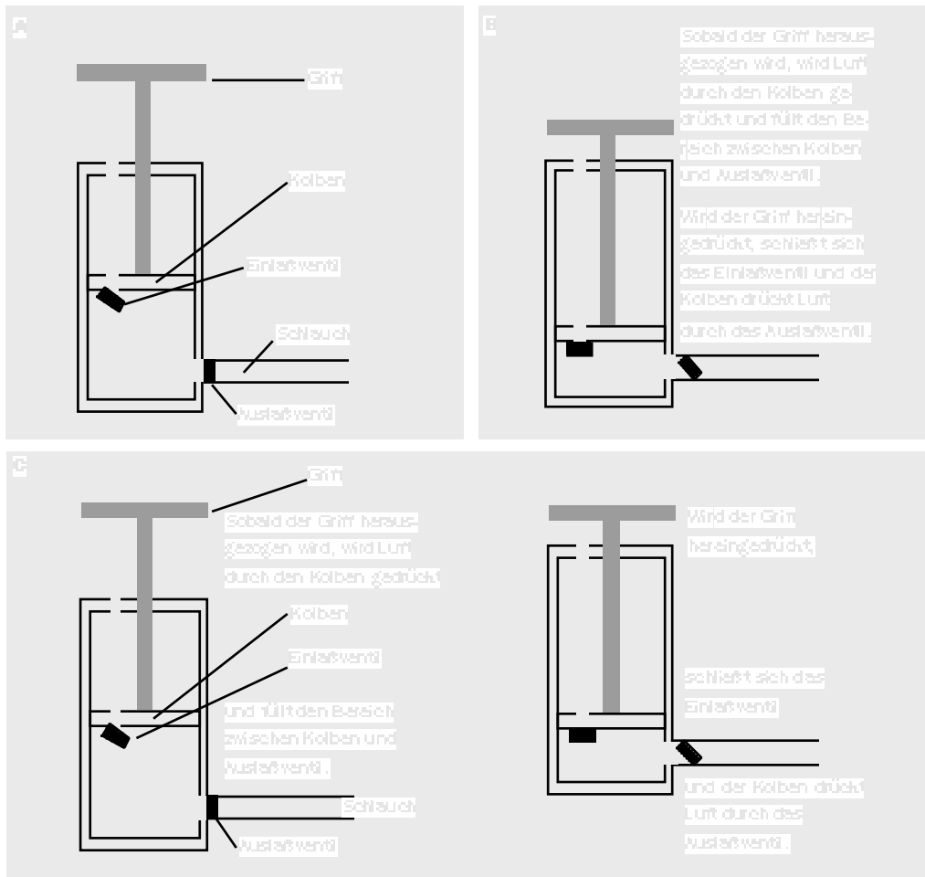
Strichzeichnungen zur Funktionsweise einer Handluftpumpe
